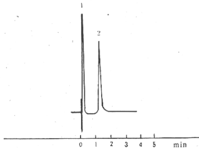
标准色谱图
