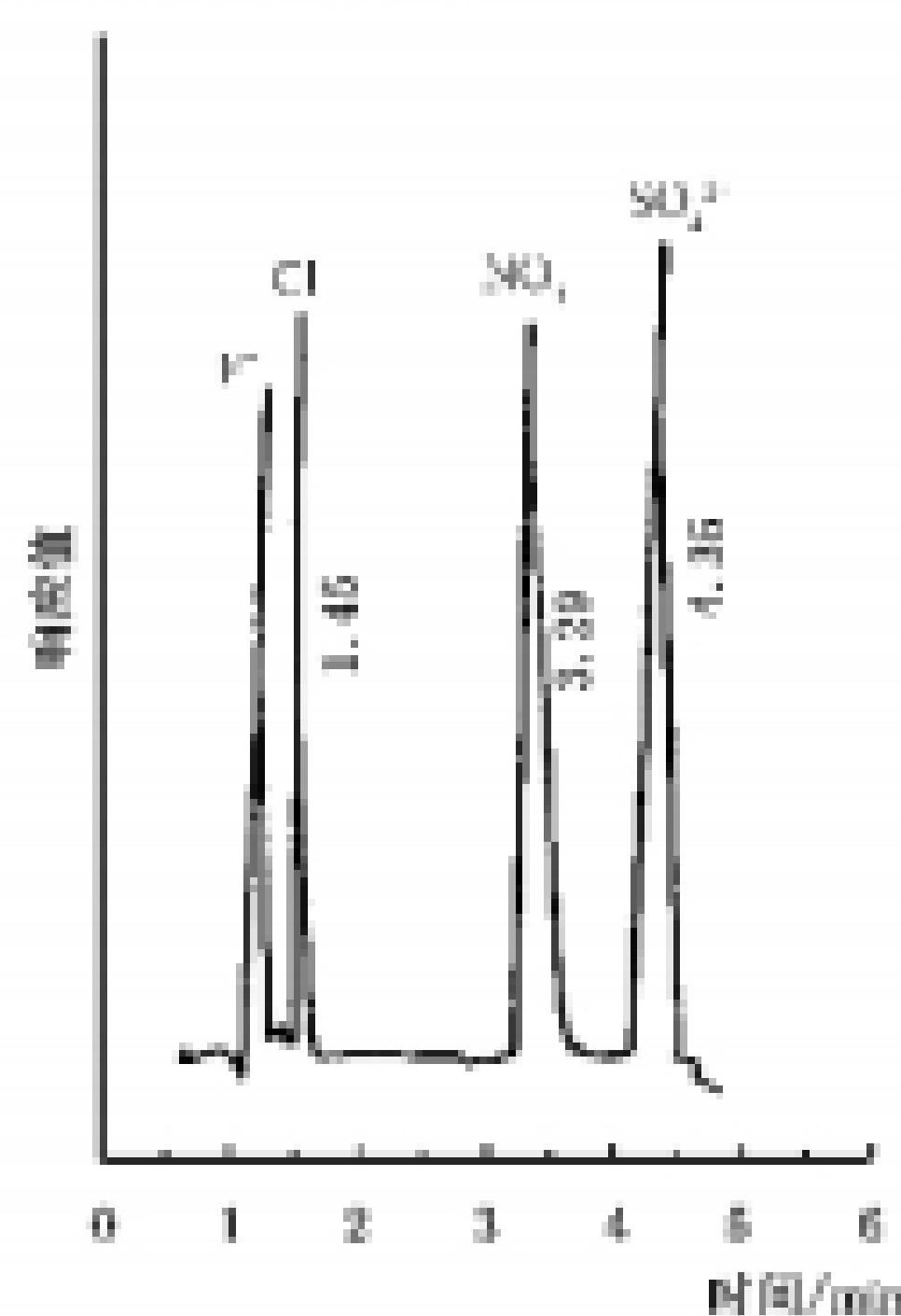
图 1 离子色谱图
